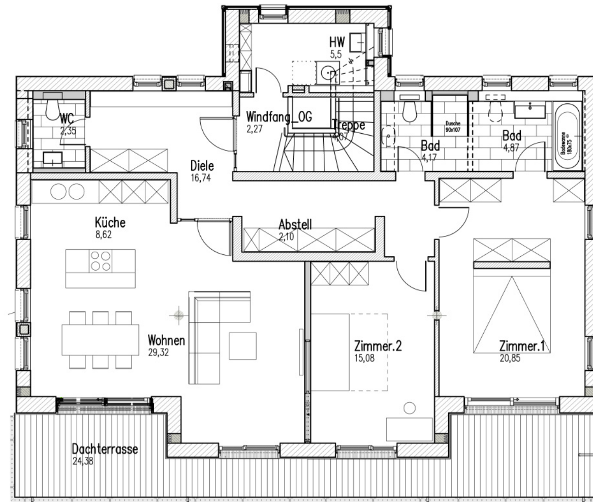
Grundriss Obergeschoß
